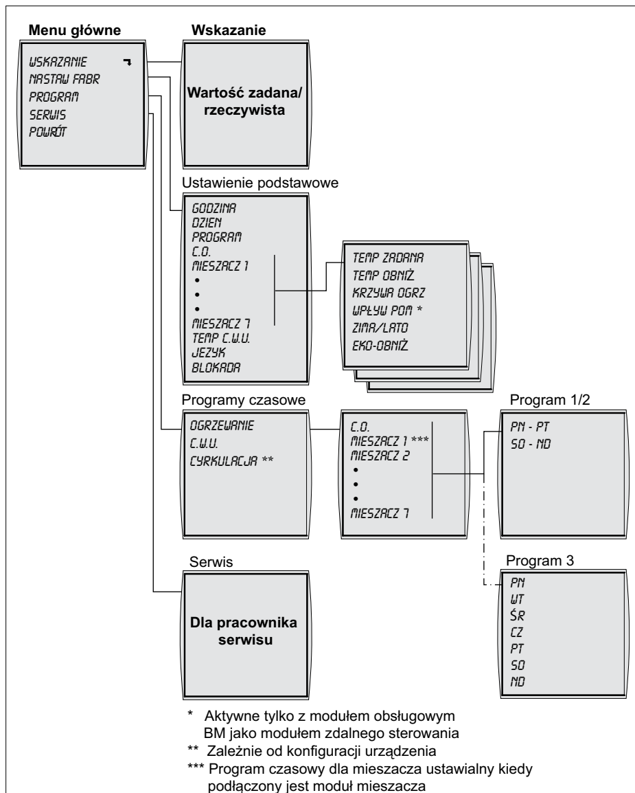
Rys. 5.1 Struktura menu modułu obsługowego BM
