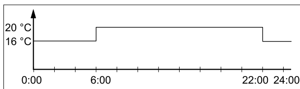
Rys. 4.2 Przykład czasu przełączania
