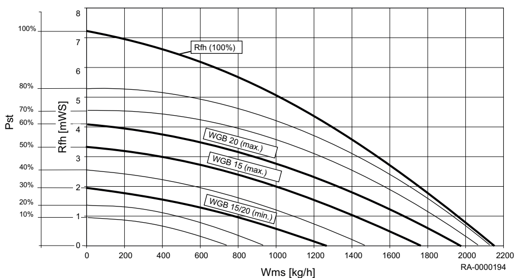
Rys.1 Łączne ciśnienie dynamiczne WGB 15 — 20
