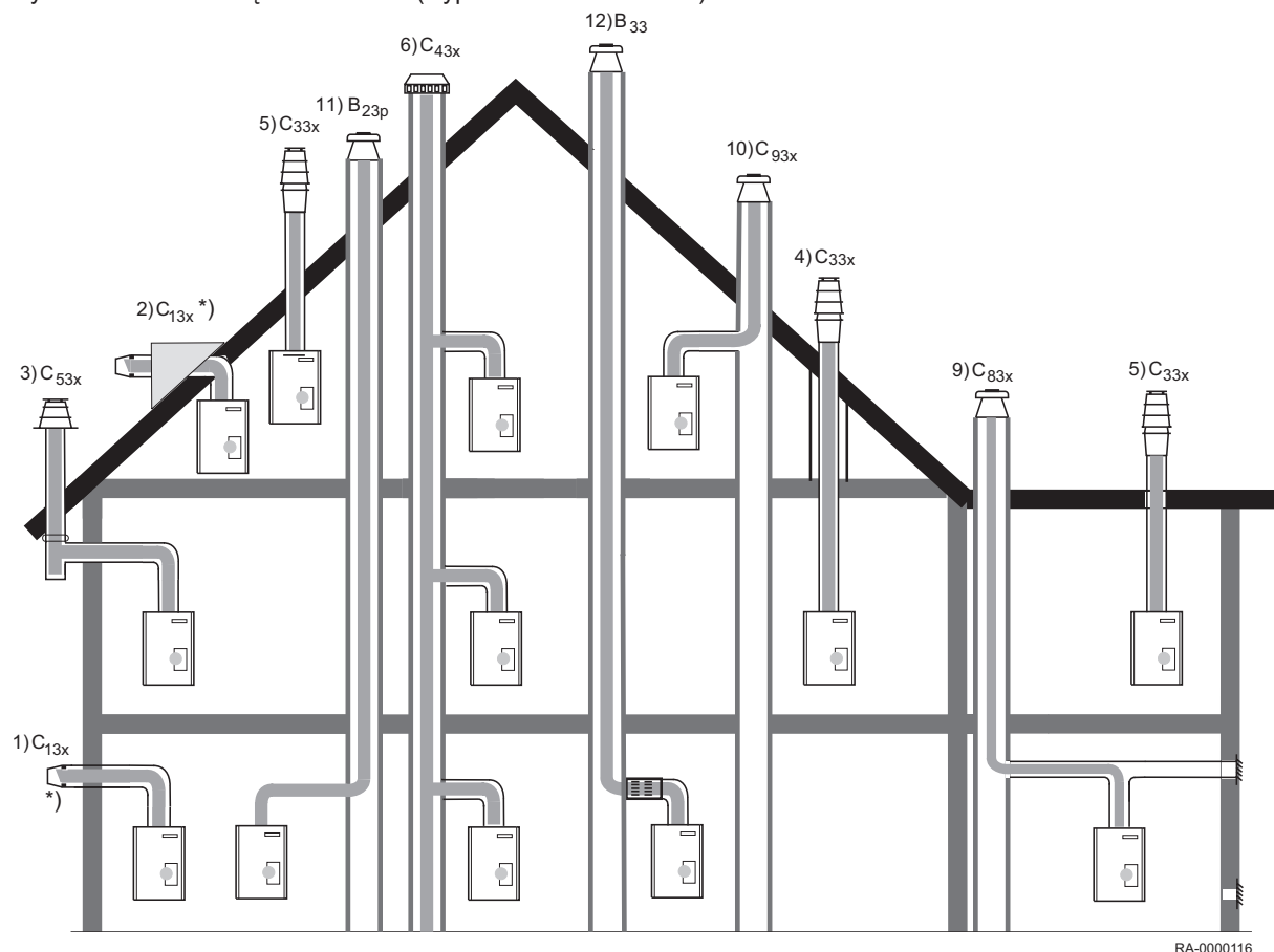
Rys.18 Możliwości łączenia z KAS (wyposażenie dodatkowe)
