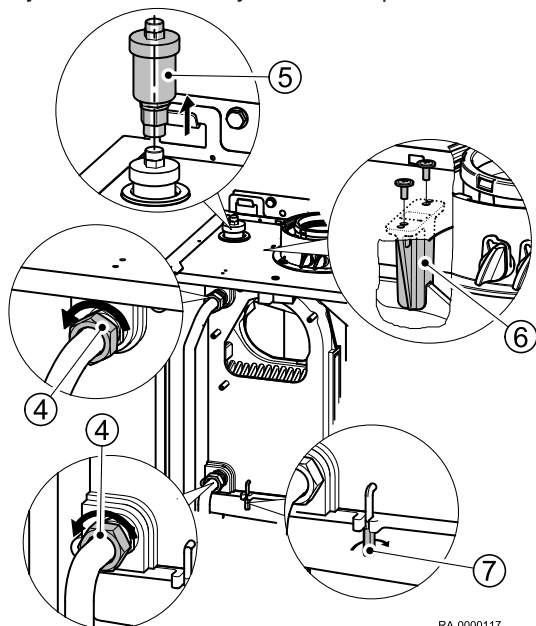
Rys.41 Demontaż wymiennika ciepła
