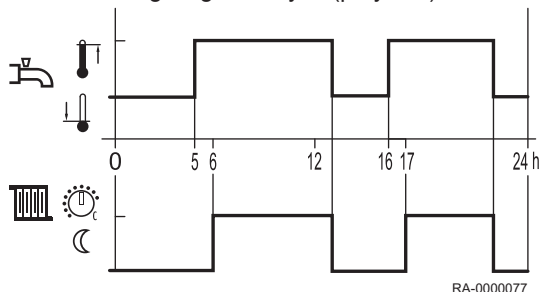
Rys.30 Odblokowywanie w zależności od programów czasowych przełączania obiegów grzewczych (przykład)
