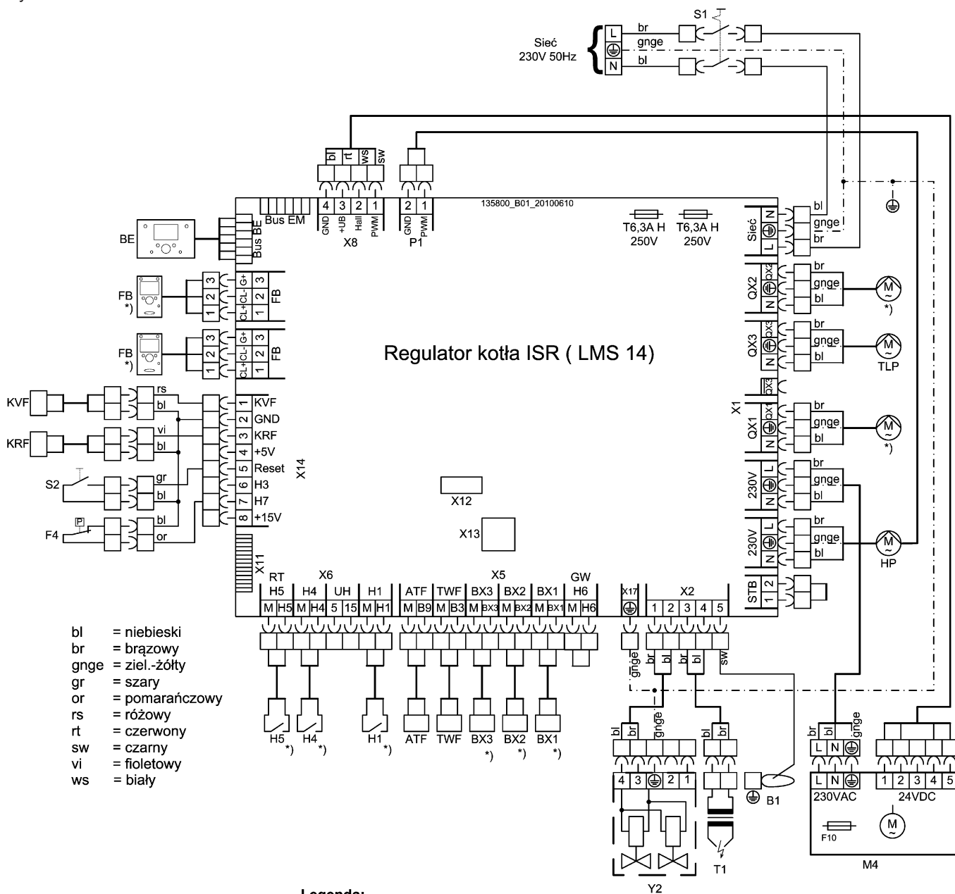
Rys.4 Schemat okablowania
