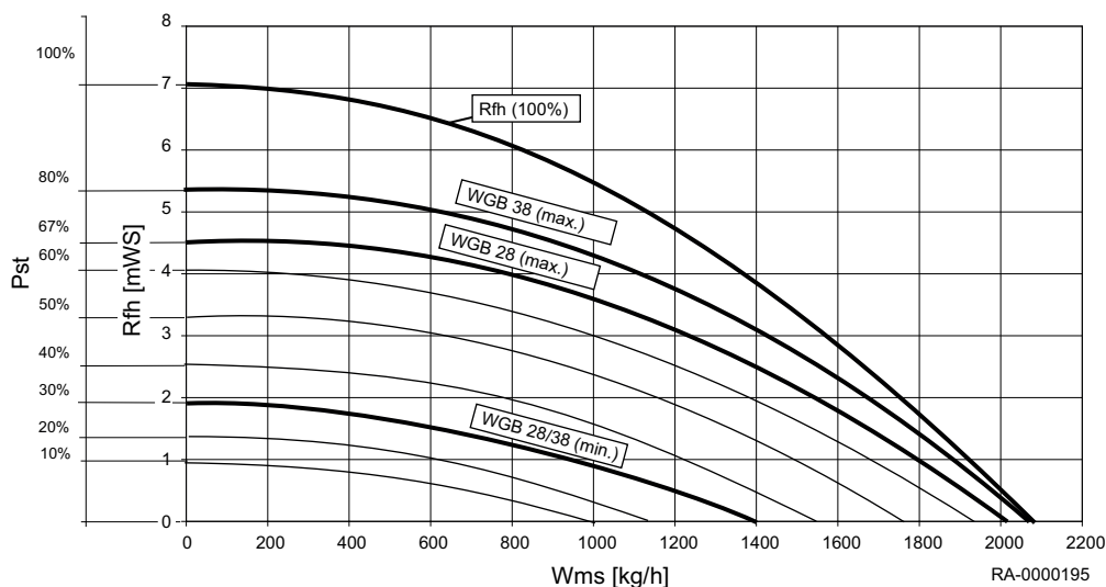
Rys.2 Łączne ciśnienie dynamiczne WGB 28 — 38
