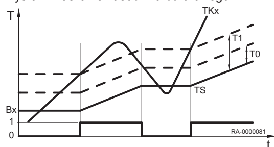
Rys.34 Zasilanie zasobnika buforowego
