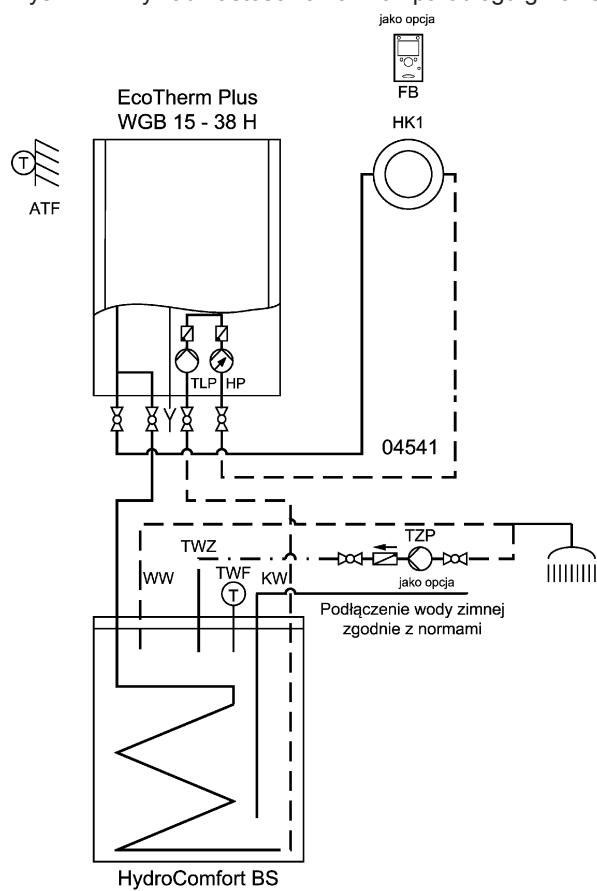
Rys.11 Przykład zastosowania: Pompa obiegu grzewczego z regulatorem pokojowym z regulacją temperatury w zasobniku
