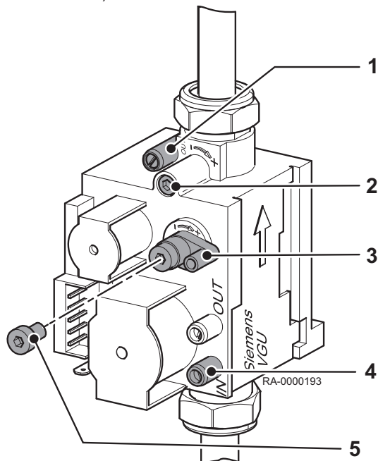
Rys.21 Zawór gazu (ustawianie ciśnienia wtryskiwacza za pomocą klucza torx T15)
