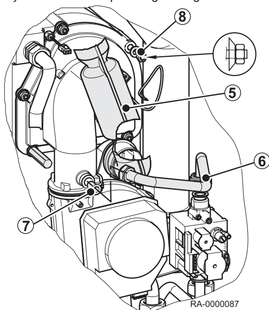
Rys.40 Demontaż palnika gazowego
