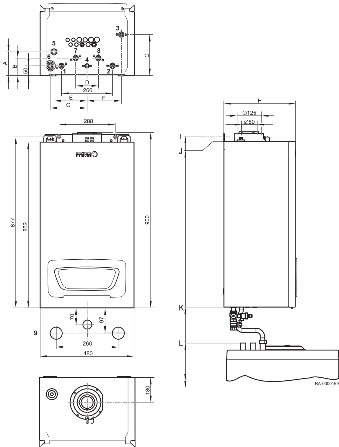
Rys.3 Wymiary i przyłącza WGB
