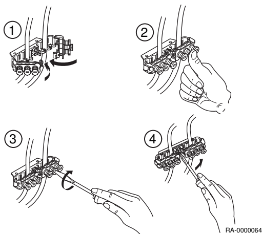
Rys.20 Zabezpieczenia przed uszkodzeniem
