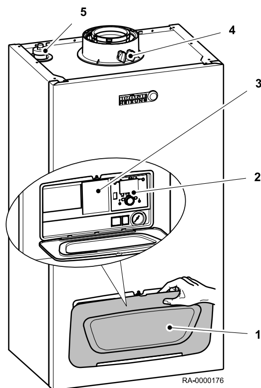
Rys.1 Schemat poglądowy WGB EVO
