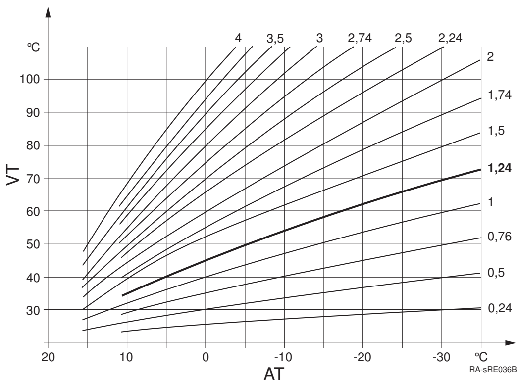
Rys.5 Krzywa grzewcza
