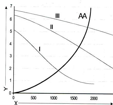
Wilo RS 15/7-3
